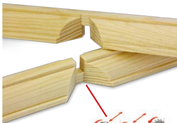
Fraisage pour croisillons
